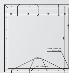
TRÄDETAJ - PLAN
