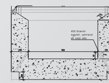
BETONGDETAJ - SEKTION A-A
